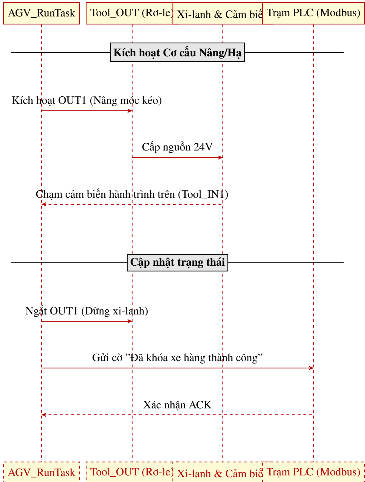
Hình 4.10 Sơ đồ tuần tự hoạt động của cơ cấu móc kéo xe hàng.
