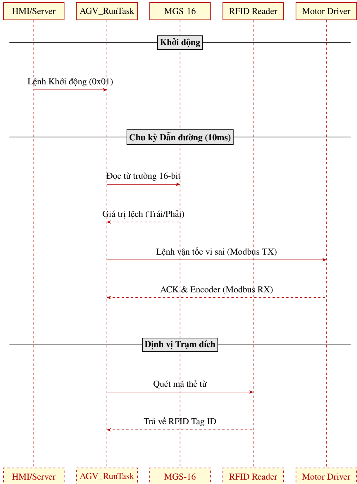
Hình 4.8 Sơ đồ tuần tự quá trình dẫn đường và nhận dạng trạm RFID.
