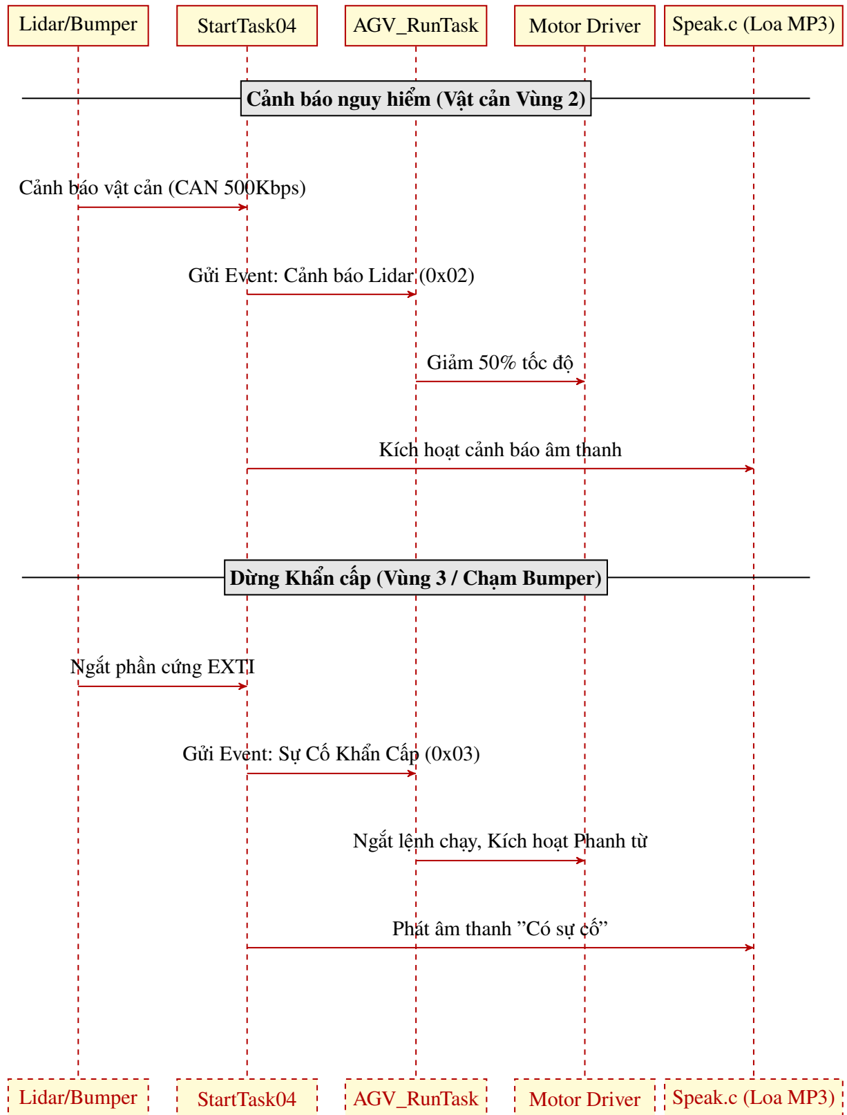
Hình 4.9 Sơ đồ tuần tự luồng giám sát an toàn và xử lý sự cố khẩn cấp.
