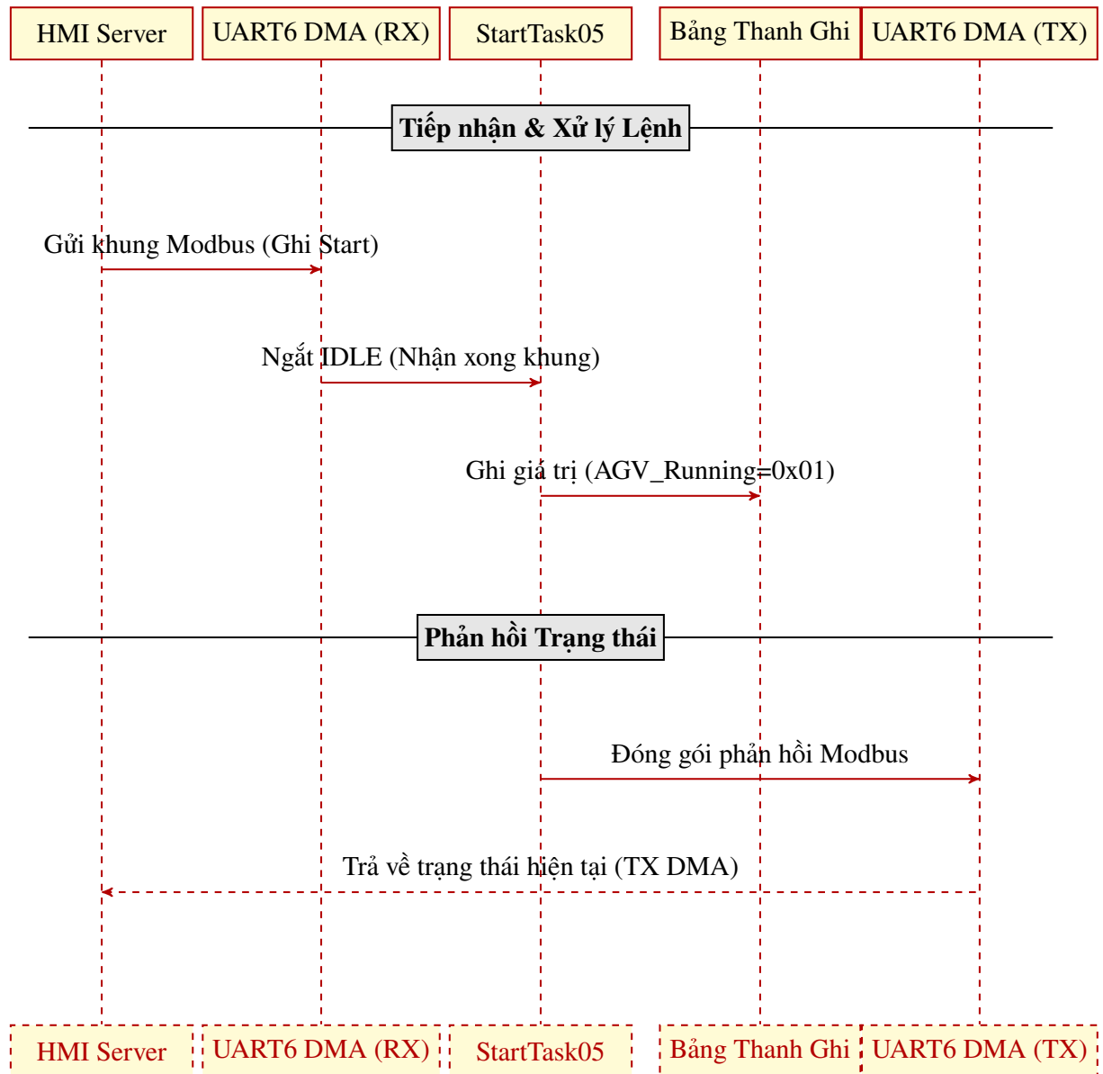
Hình 4.12 Sơ đồ tuần tự giao thức truyền thông Modbus RTU.
