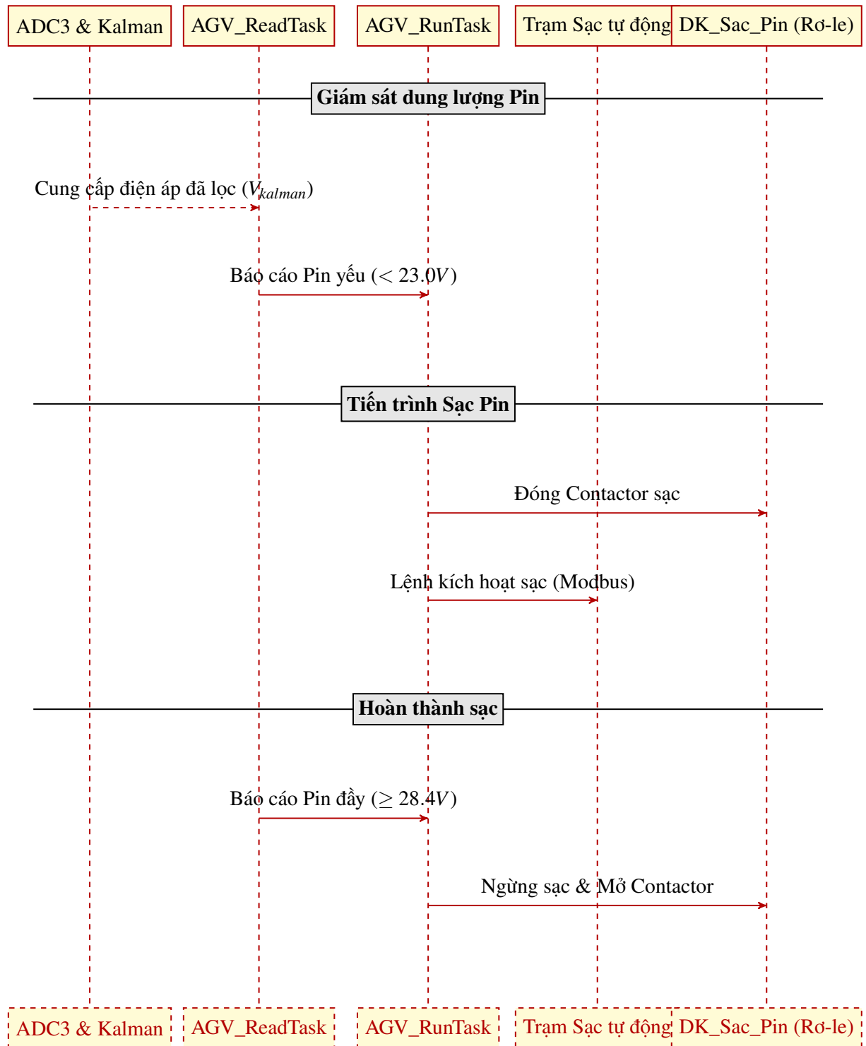
Hình 4.11 Sơ đồ tuần tự quá trình giám sát Pin và sạc tự động.
